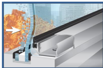
La zona di movimento incorporata nel FrameGard assorbe l'energia permettendo alla pellicola di allungarsi. La superficie a grip tiene la pellicola in posizione.
